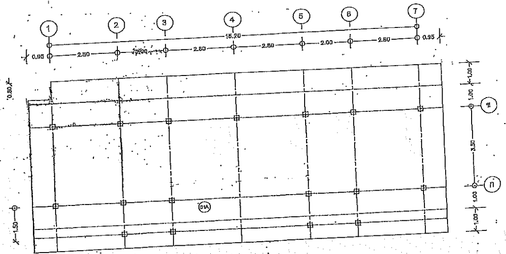
แปลนตำแหน่งประตู (แก้ไข) บ้านหลังที่ 1 ชั้นล่าง ด้านหน้า
