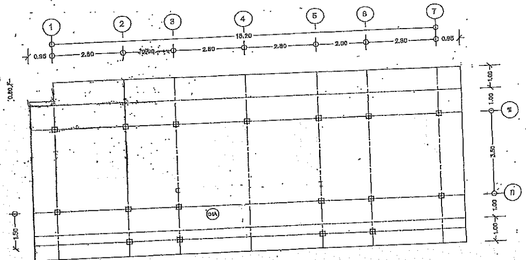
แปลนตำแหน่งประตู (แก้ไข) บ้านหลังที่ 4 ชั้นล่าง ด้านซ้าย
